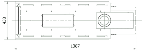
B-B (1 : 10)
